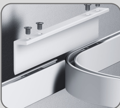
Verbindingsbrug
