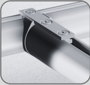
T-Verbinder
