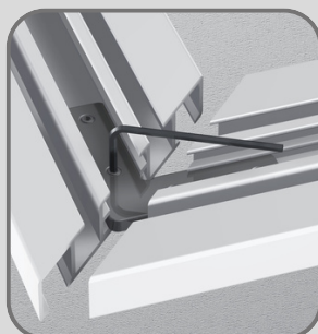
Hoekverbinder
