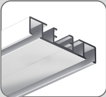
Gordijnrail A6740
