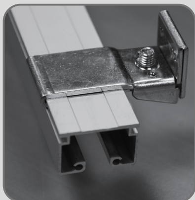
Wandsteun
