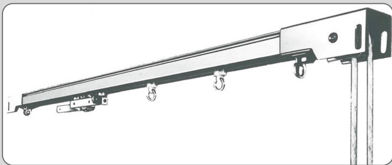
Koordebediende rail A6520 geassembleerd
