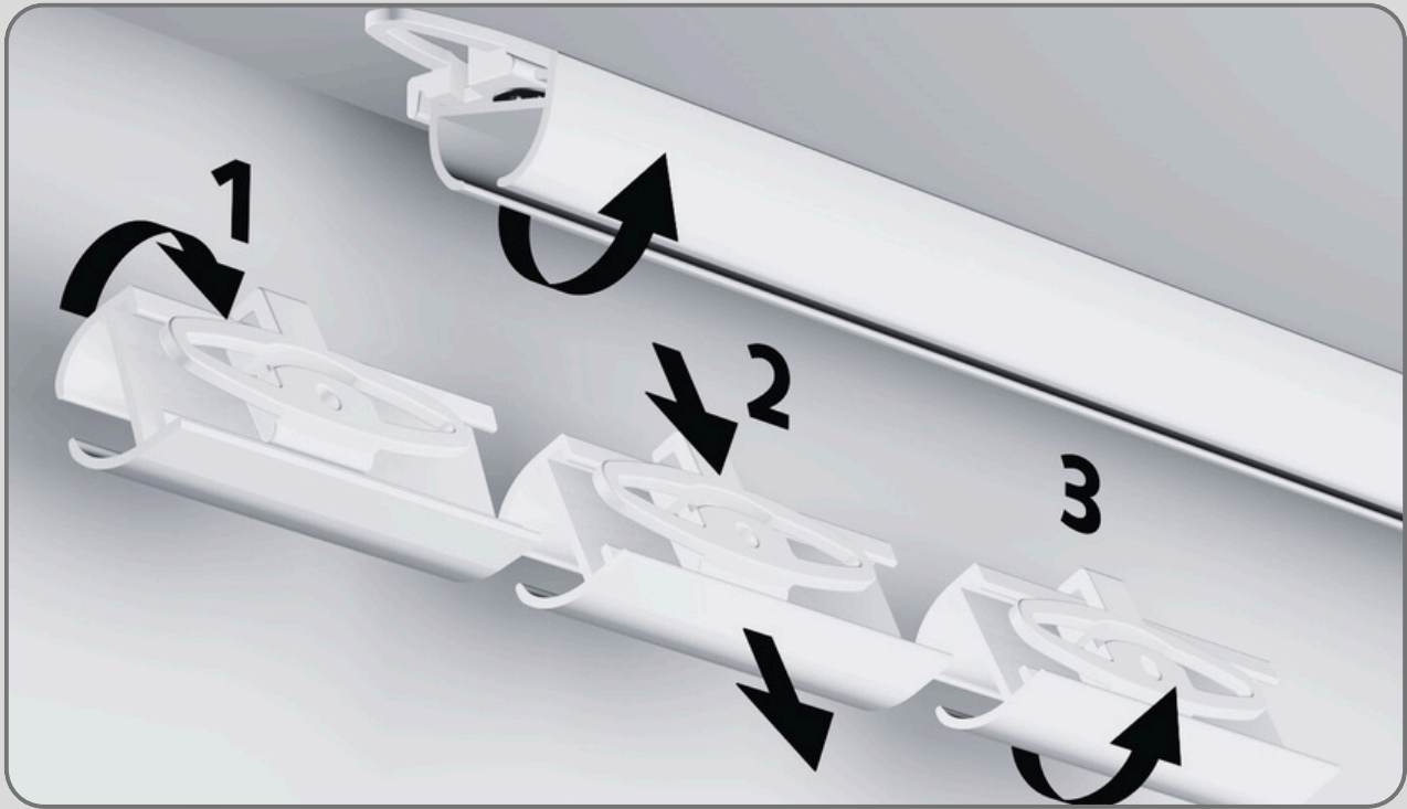
Montage plafondclip
