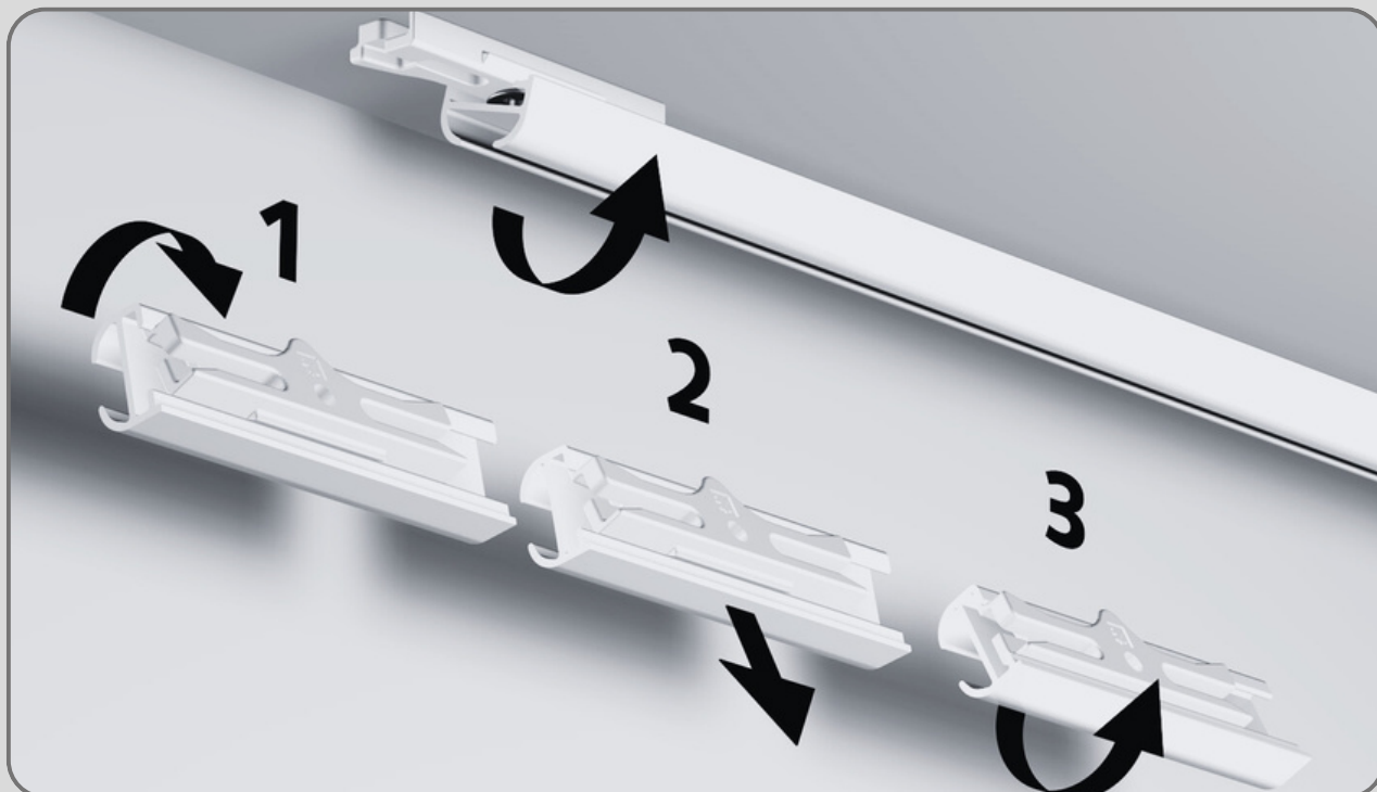
Montage plafondclip
