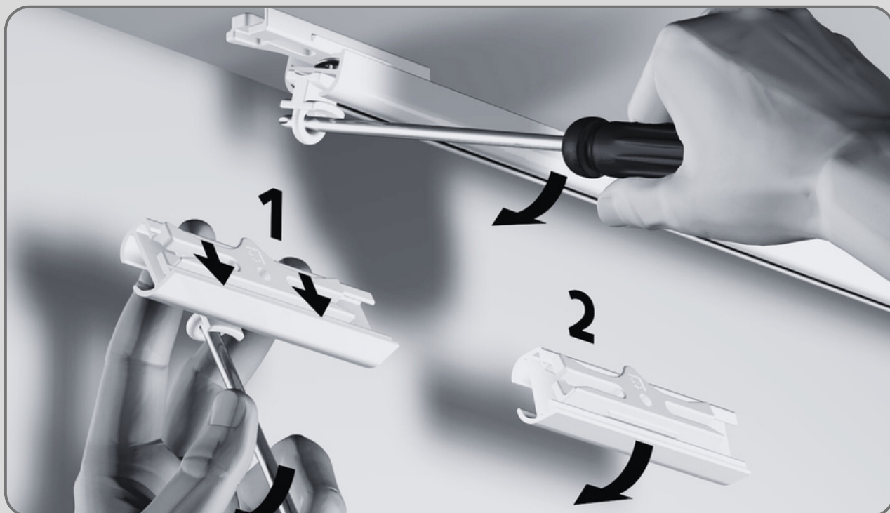
Demontage plafondclip
